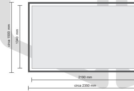
BUITENZIJD | rechterzijde en linkerzijde (boven) Signing spandoeken in buizenframe (montage met elastieken) op aanvraag doekmaat: 2190x1340mm
